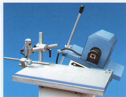
Наклон на пробивната глава Beidseitig schwenkbares Bohraggregat Tilting of the boring head
