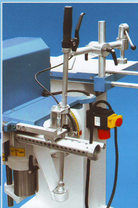
Линеал въртящ Gehrungsanschlag Miter fence
