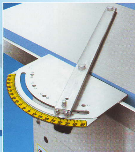
Линеал въртящ Gehrungsanschlag Miter fence
